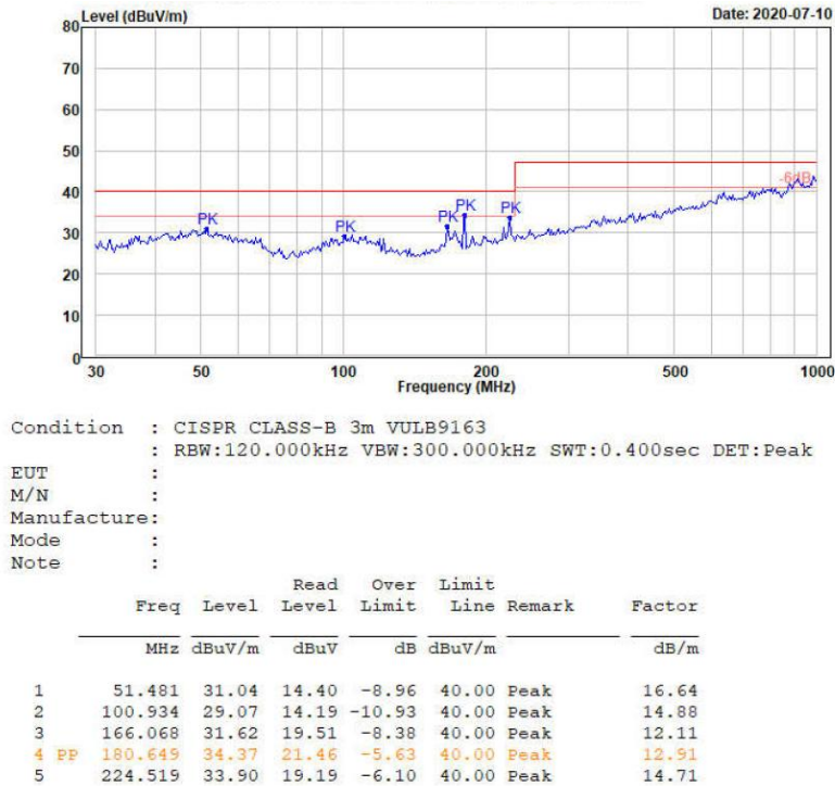
图 4-5 RE 测试水平方向
