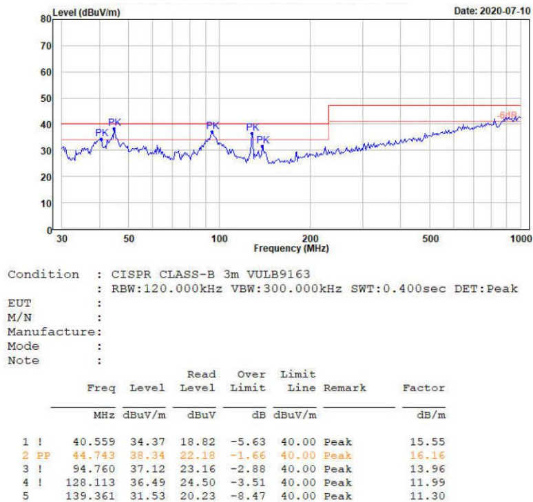
图 4-6 RE 测试垂直方向
