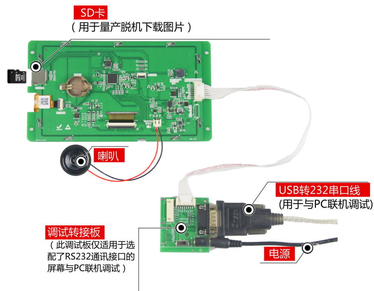
图 1-5 调试工具图
